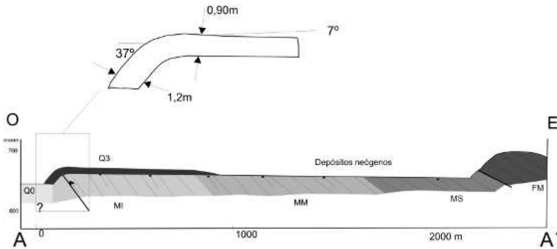
Figura 4: Perfil A-A' (indicado en la figura 2) en el que se advierte la flexura monoclinal, presente, en el sector occidental, en depósitos correspondientes a la Unidad Q3. MI: miembro inferior (gris claro), MM: medio, MS: superior y FM: Formación Mogotes.
