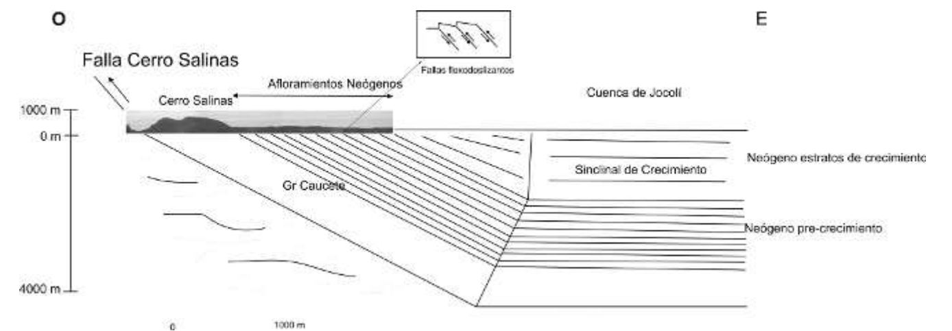
Figura 7: Esquema estructural basado en datos e interpretaciones de Vergés et al. (2007), mostrando la posición del sinclinal que incluye la estructura del área de estudio y la estratificación terciaria participante.
